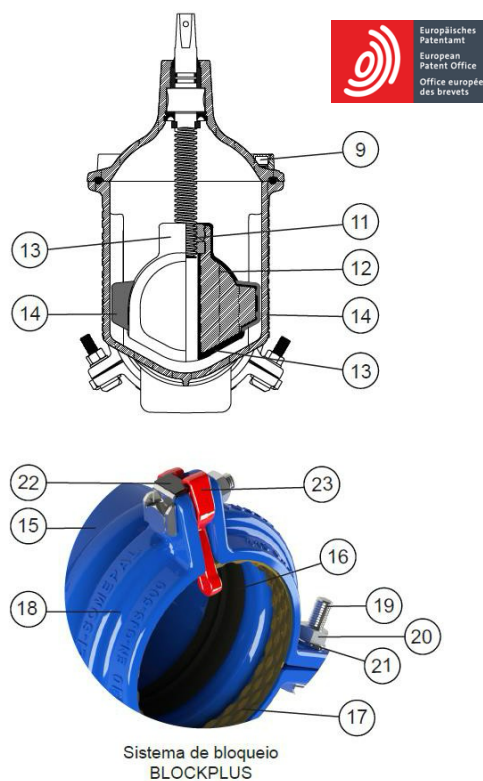
Figura 3 – Válvula de cunha elástica PE/PVC Nexus Blockplus [ref. 01.410]
