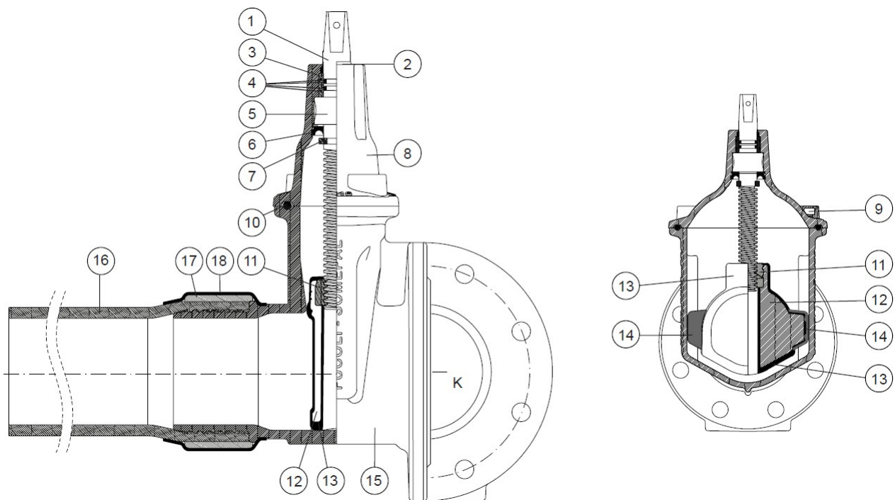
Figura 4 – Válvula de cunha elástica flange/extremidade PE Nexus [ref. 01.511]
